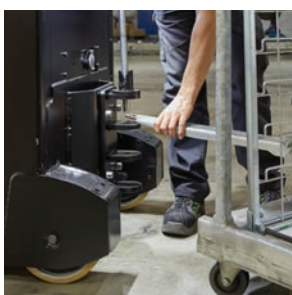
Сцепное устройство с ручным управлением
